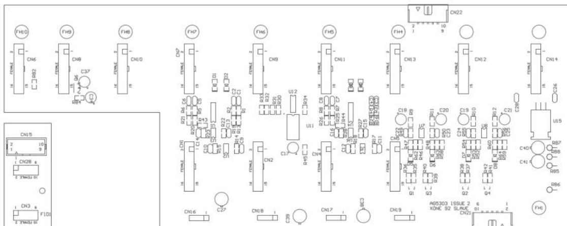
004-244 PCB ASSY XONE:92 SLAVE
