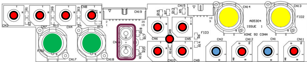
003-142 PCB ASSY XONE:92 CONN
